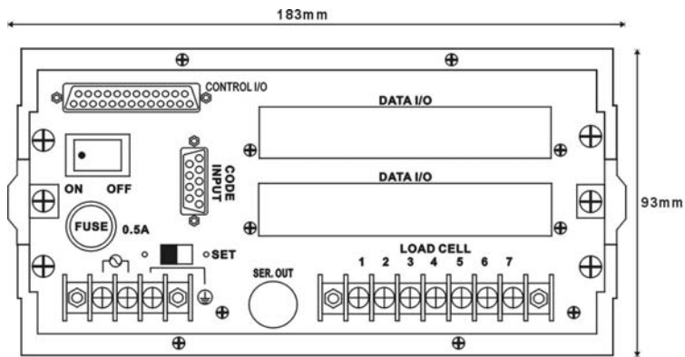
後視圖
